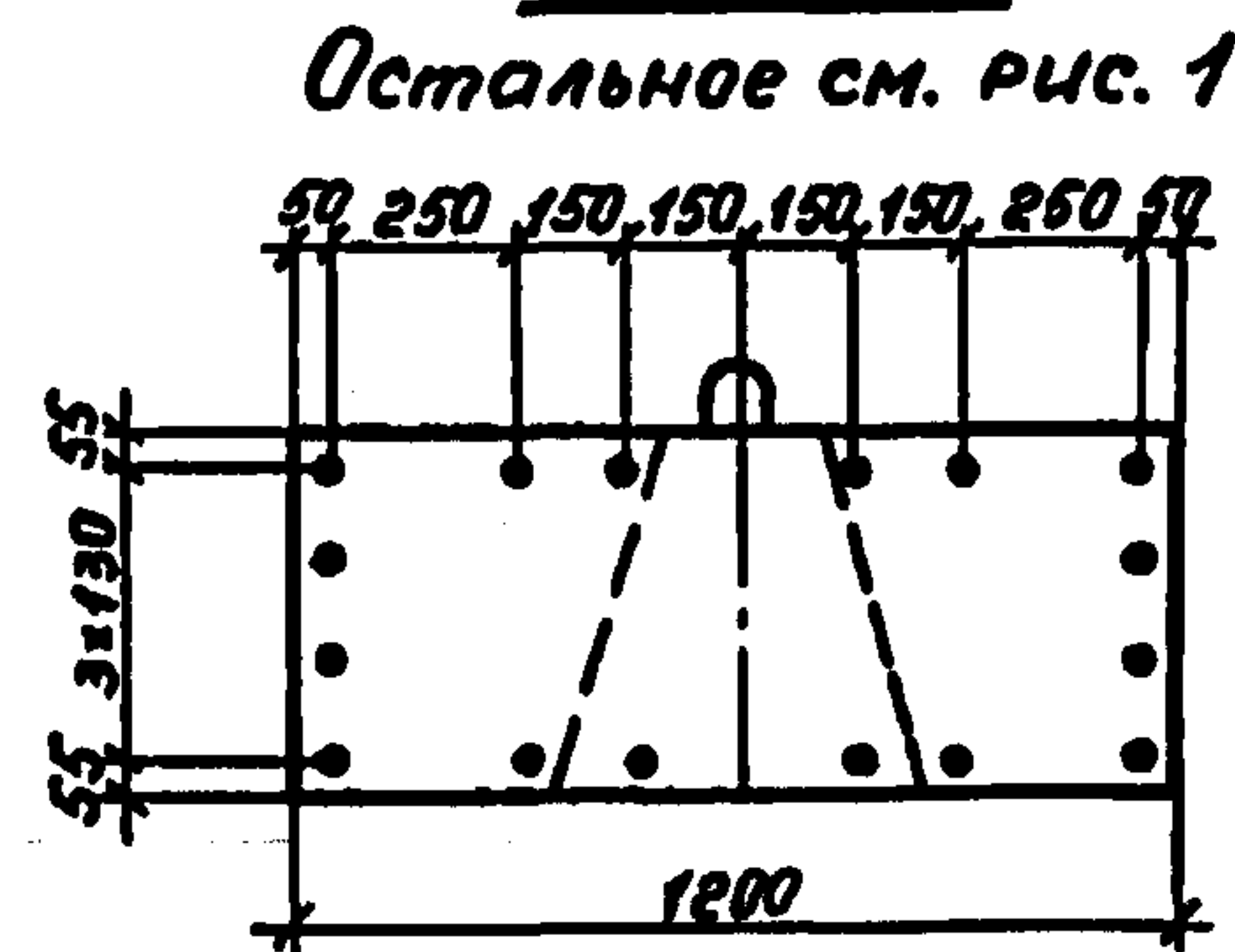
Вид 2-2
