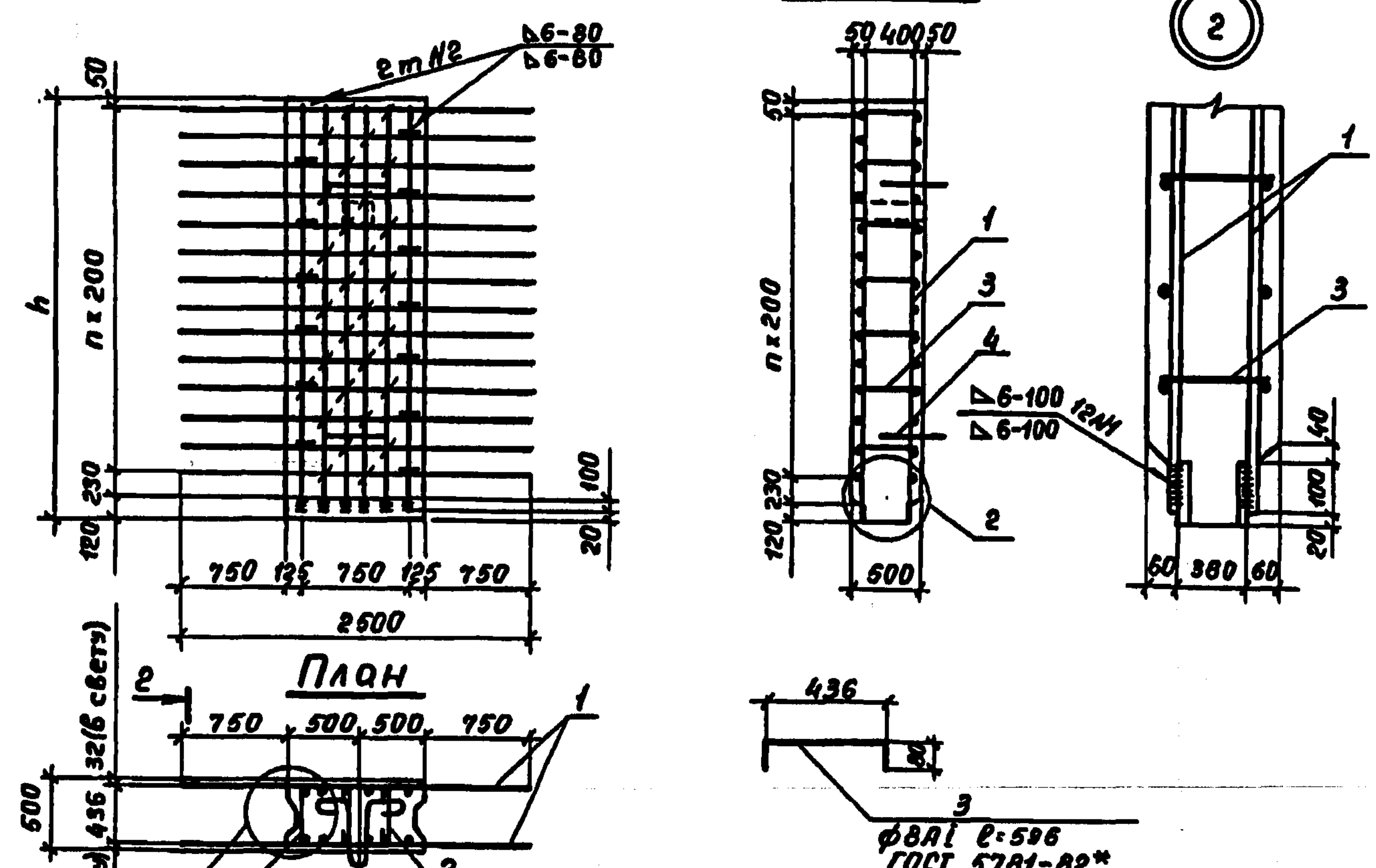
Схема армирования Вид 2-2
