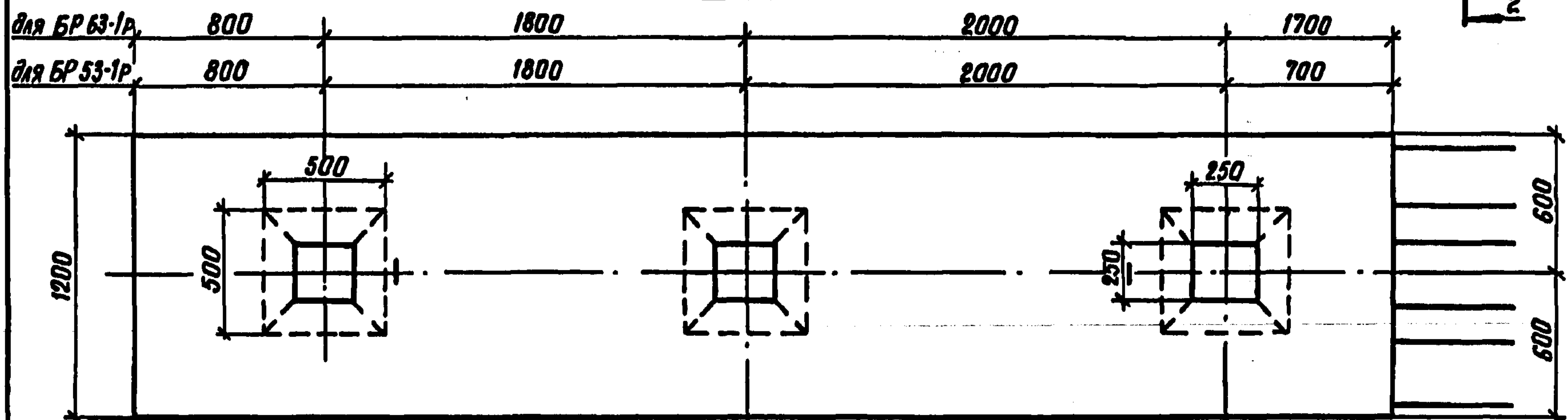
Схема армирования
