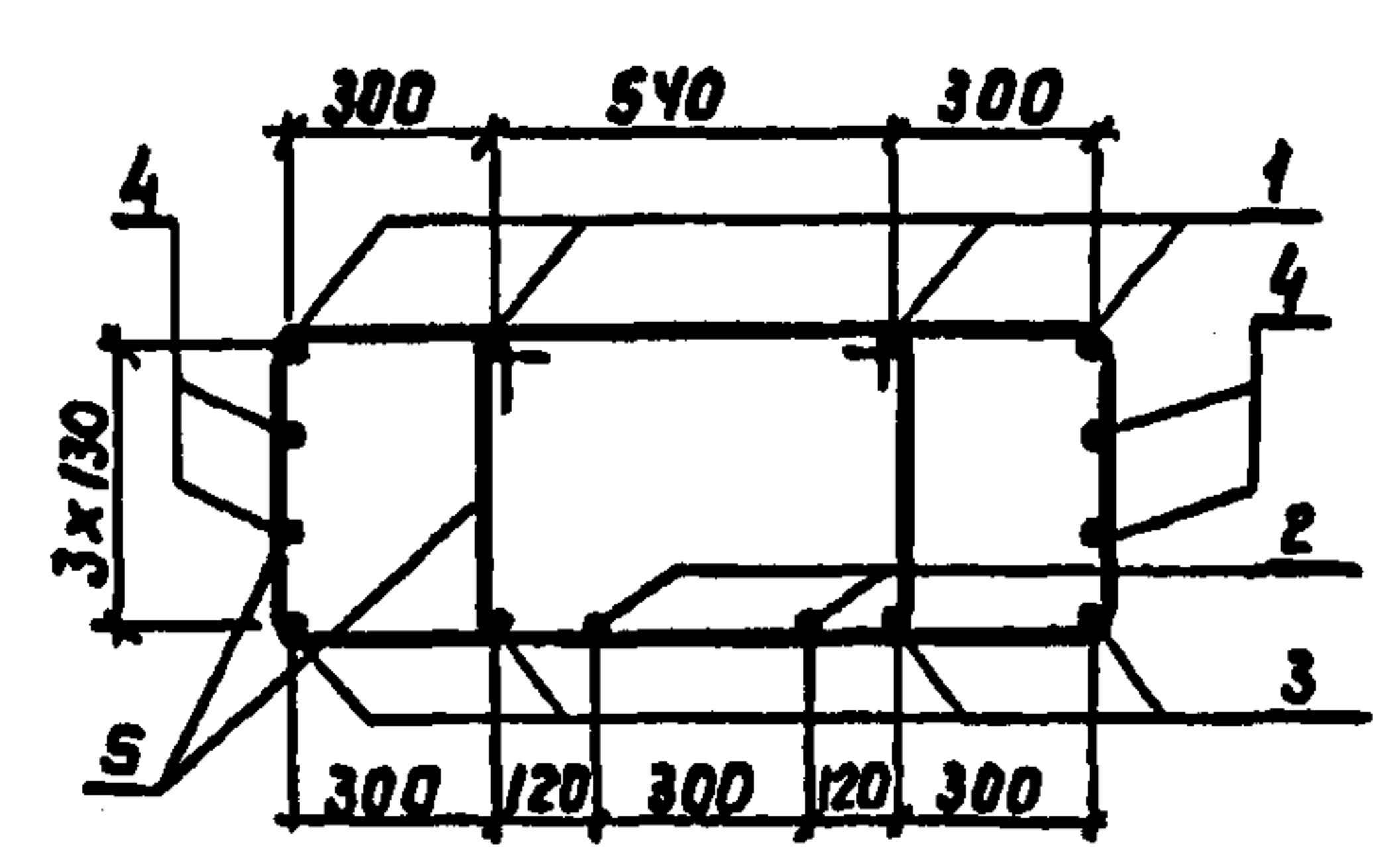
Сечение 1-1
