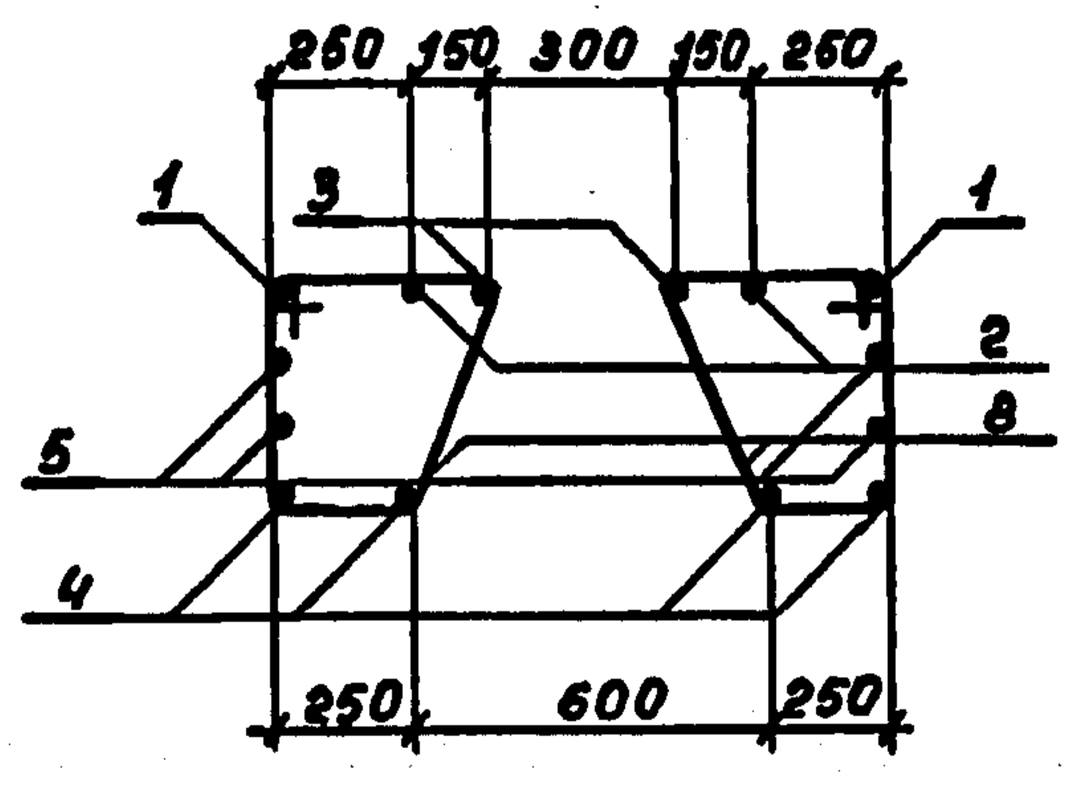
Сечение 2-2
