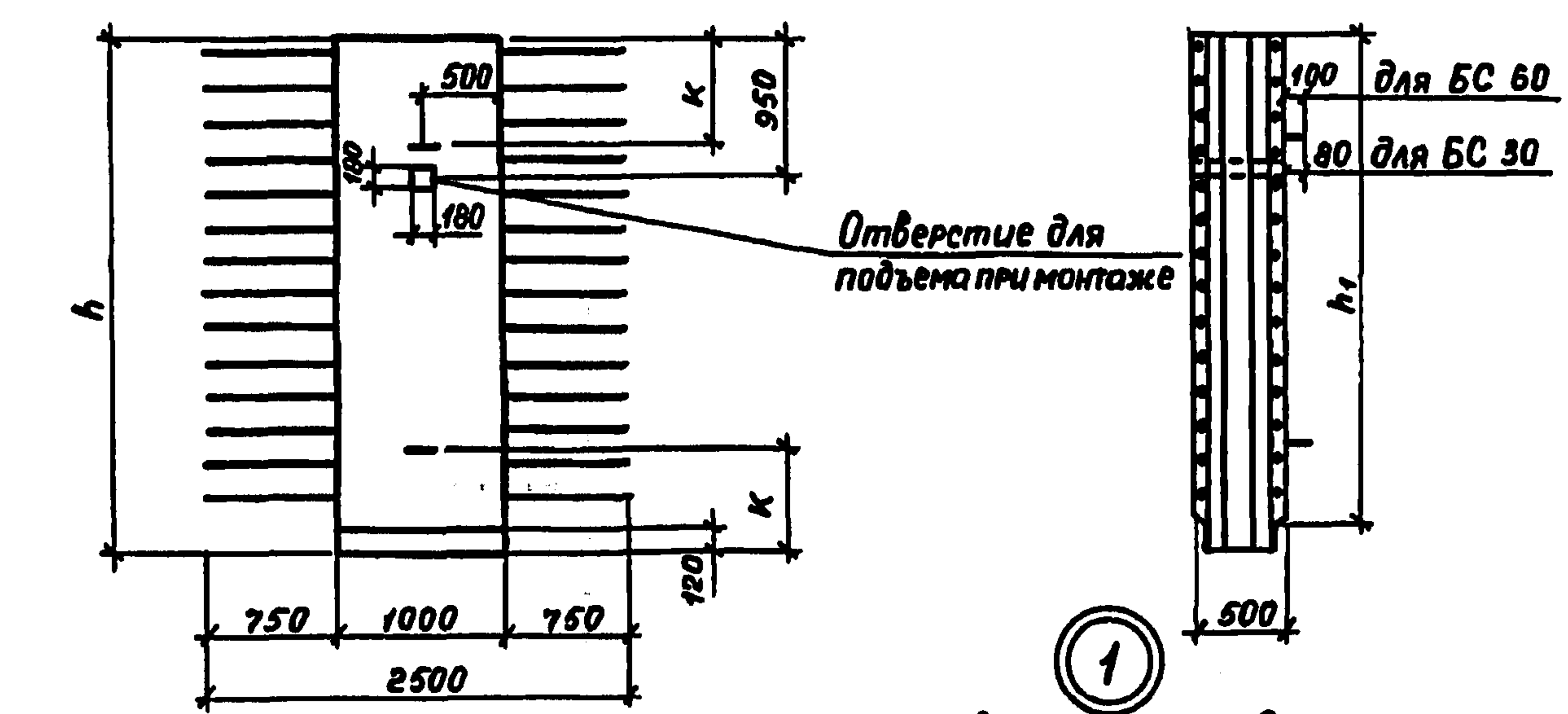
Вид 1-1
