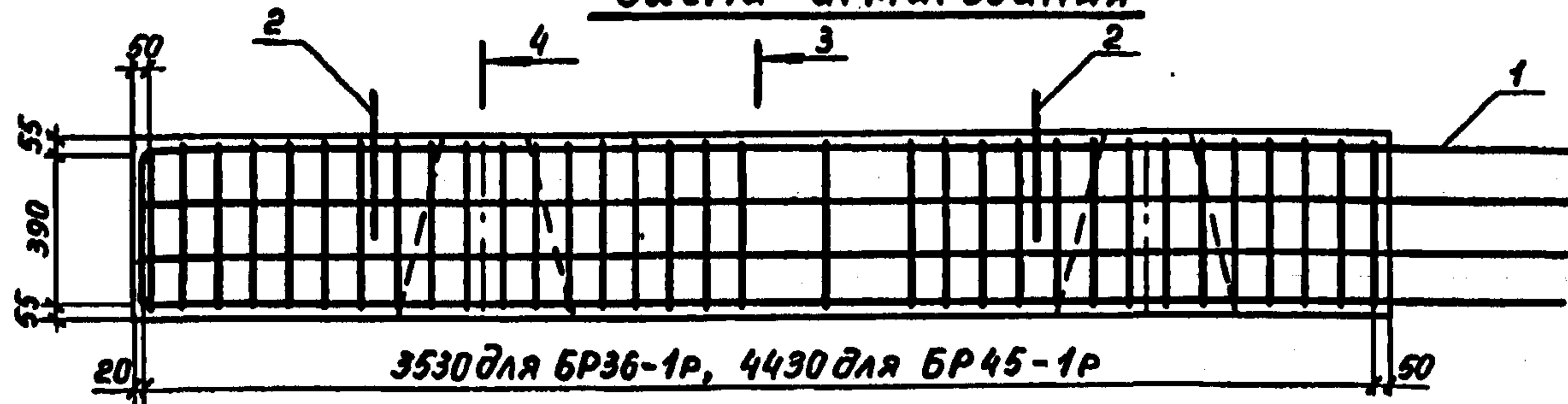
Сечение 3-3
