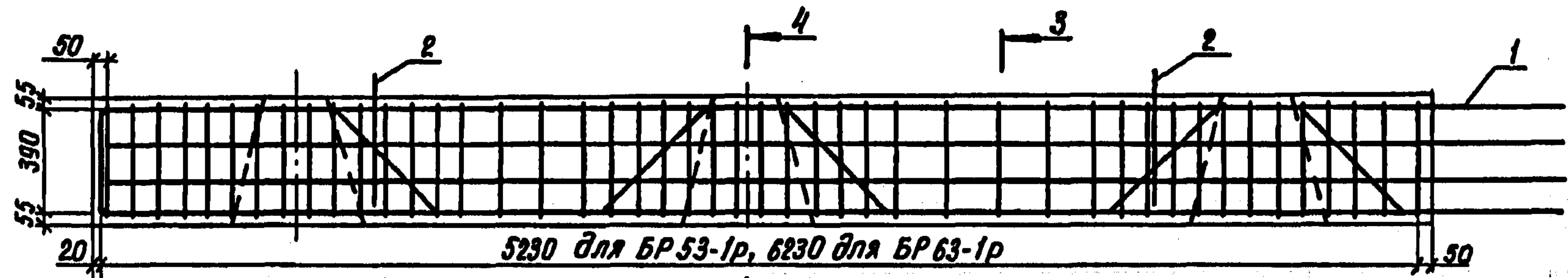
Схема армирования
