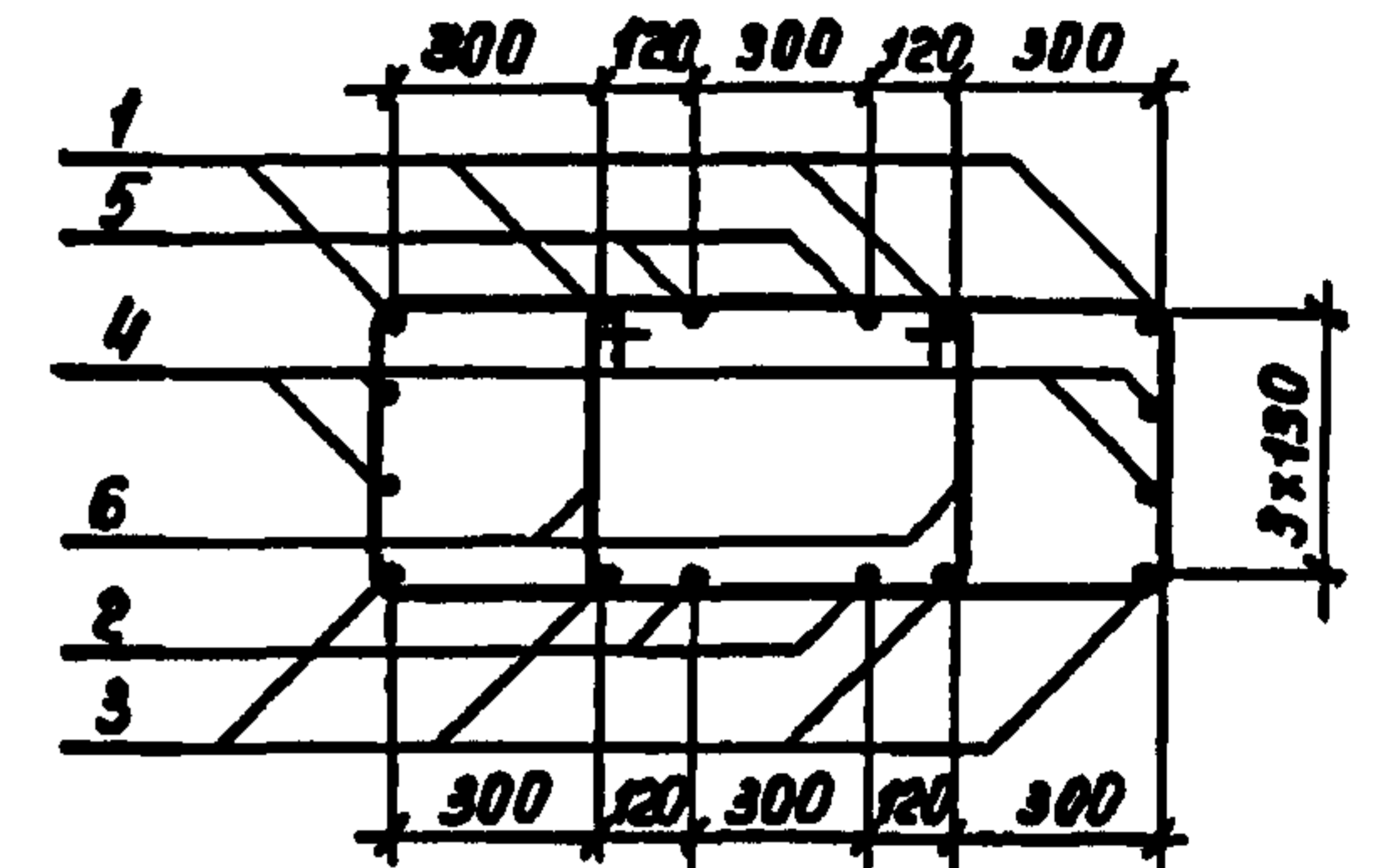
Сечение 3-3 Остальное см. рис. 1
