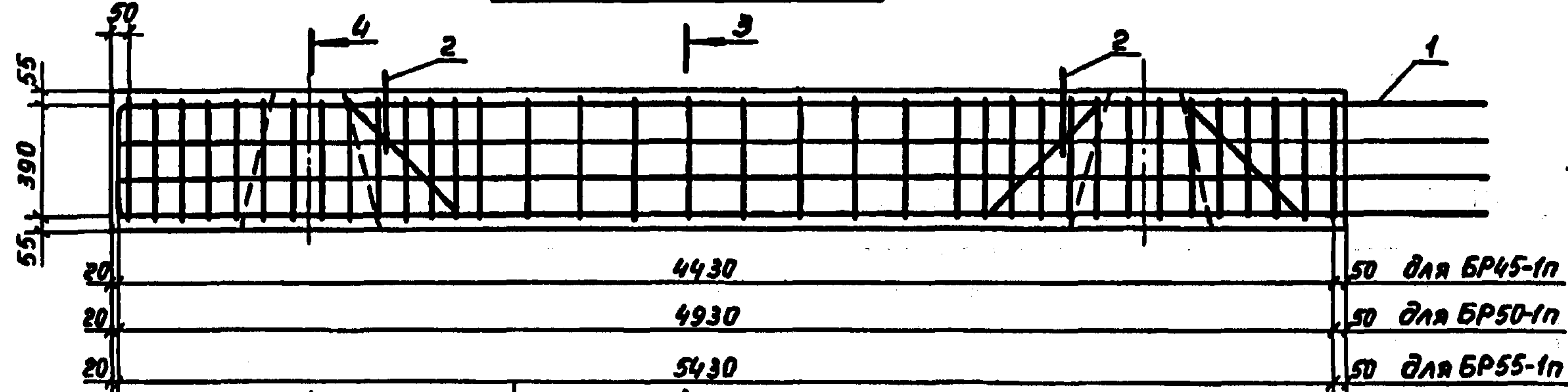
Схема армирования
