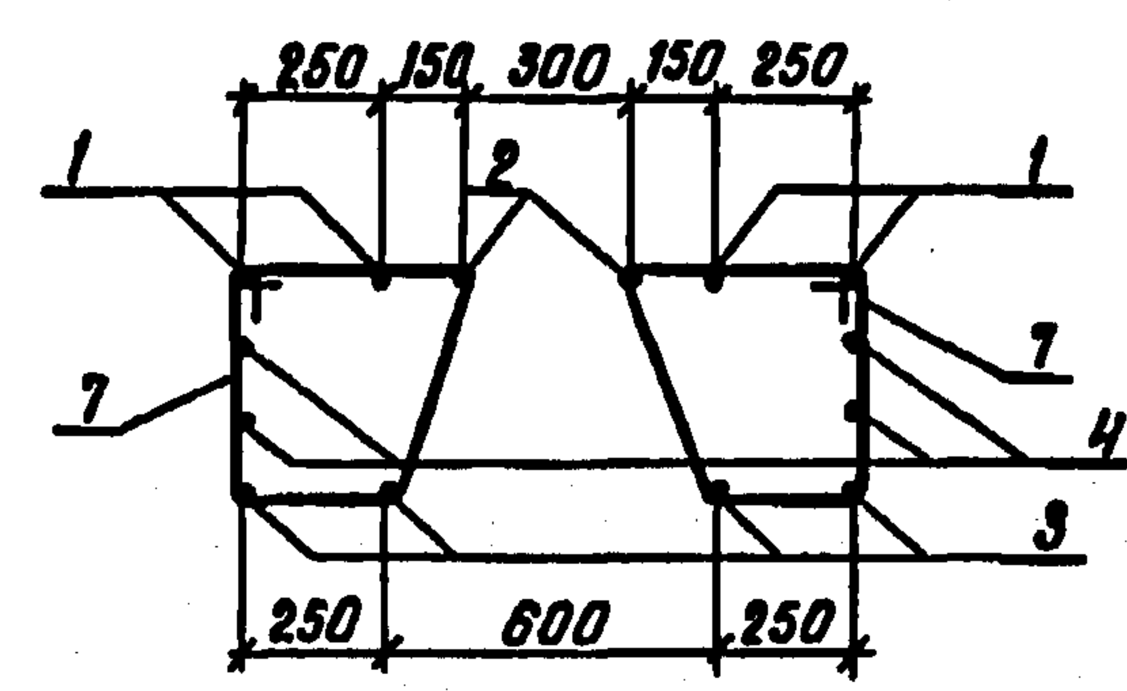
Сечение 2-2
