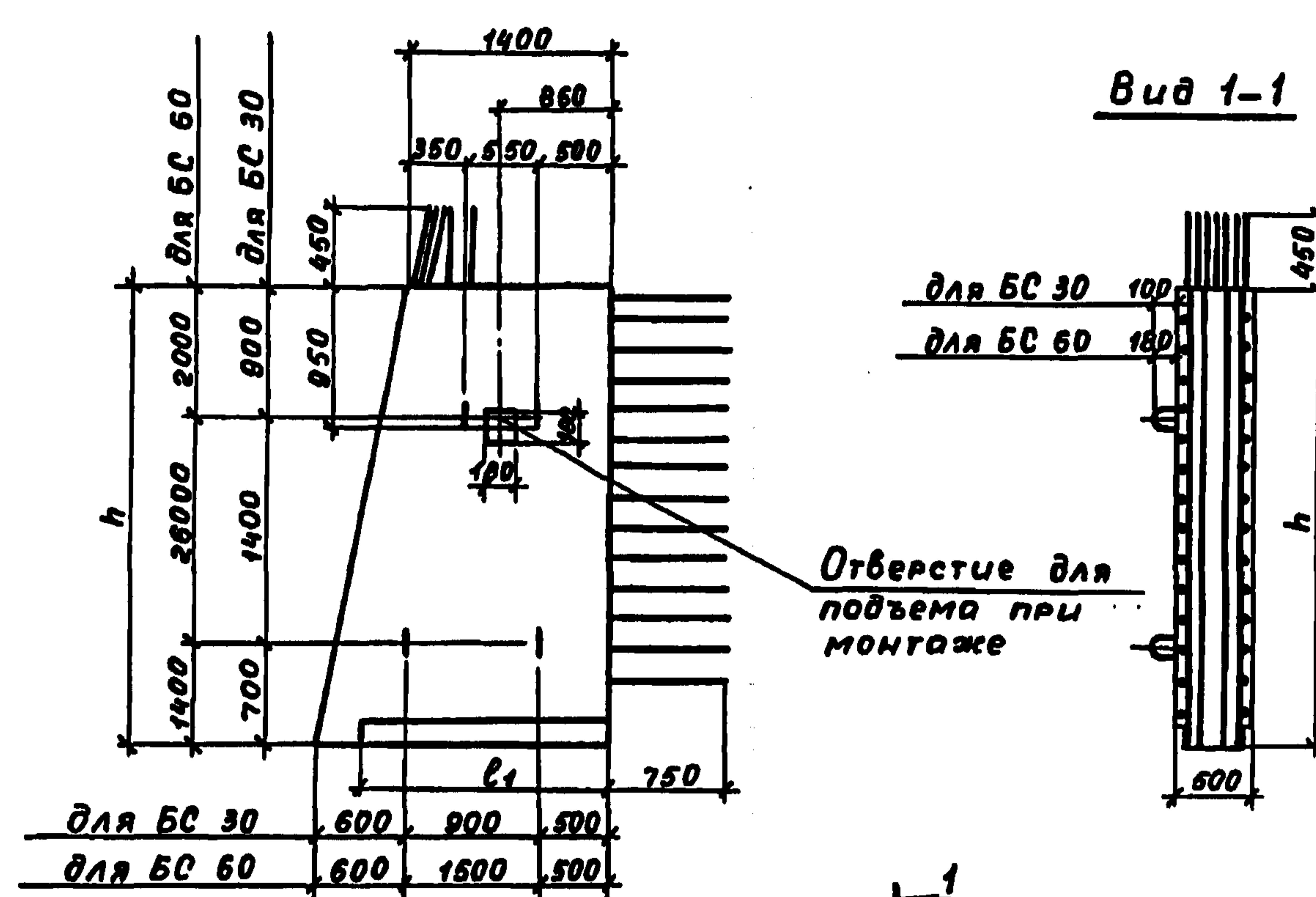
План
