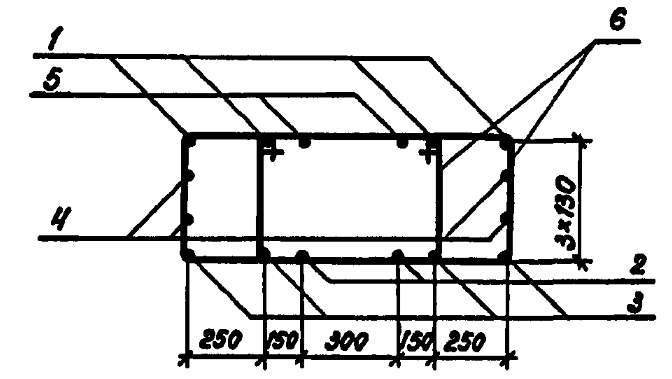
Рис. 2 Сечение 3-3 Остальное см. рис. 1
