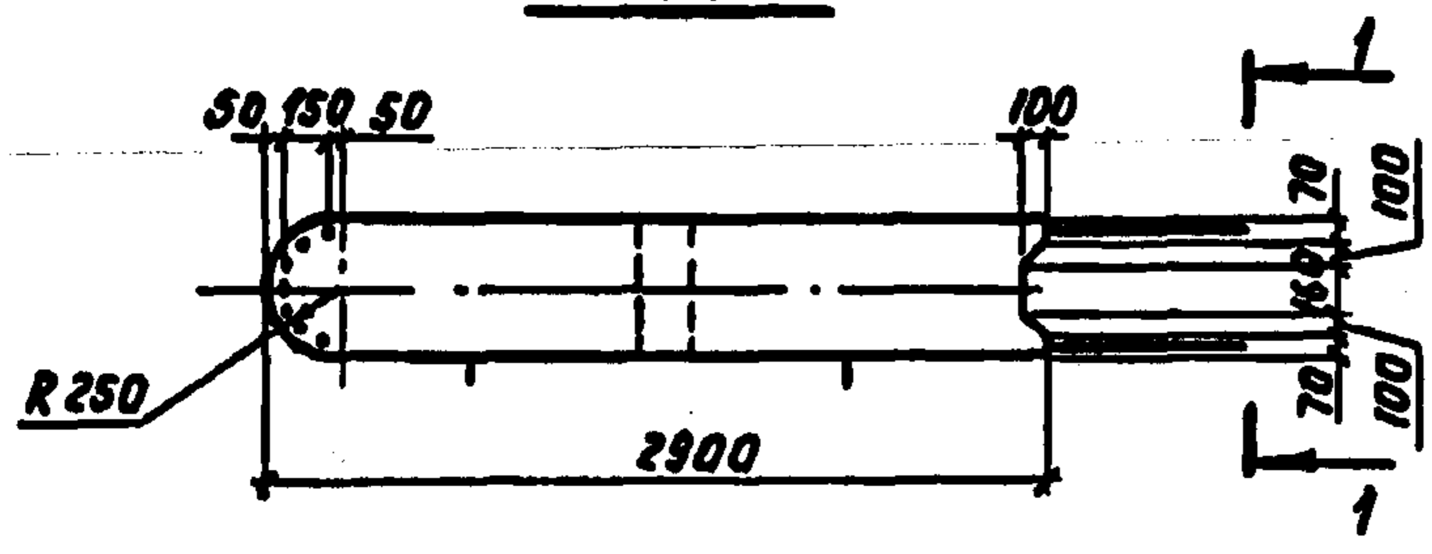
План
