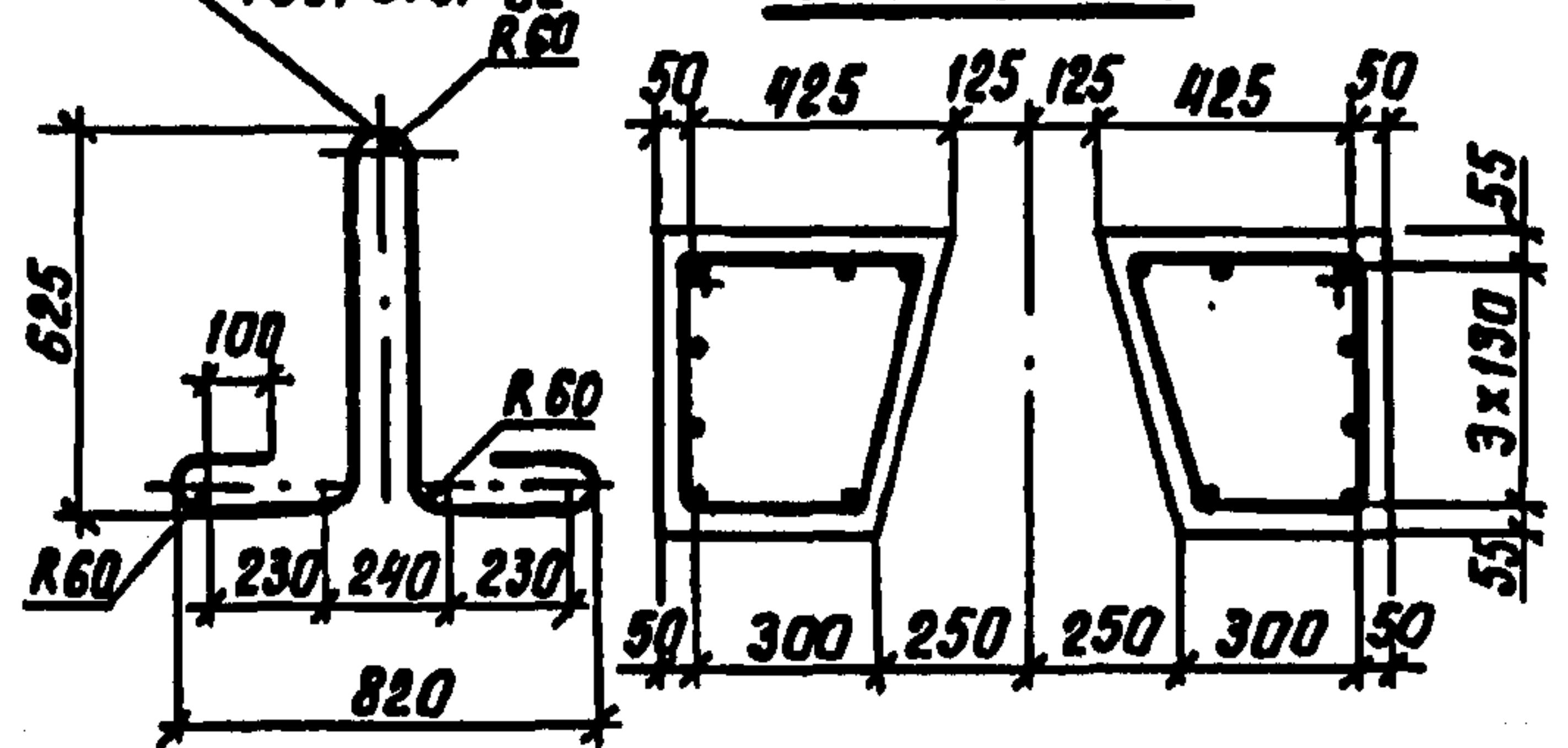
Сечение 4-4
