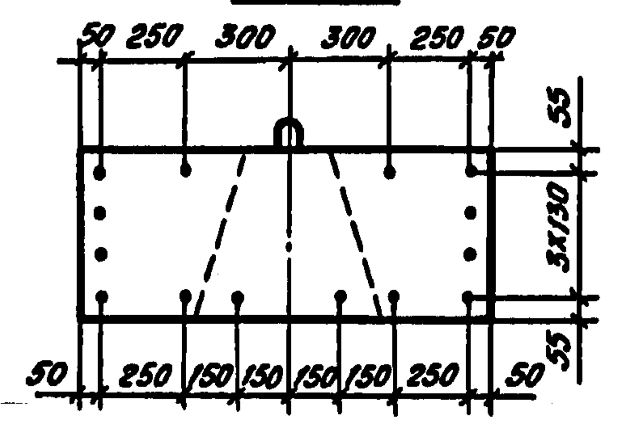
Вид 2-2
