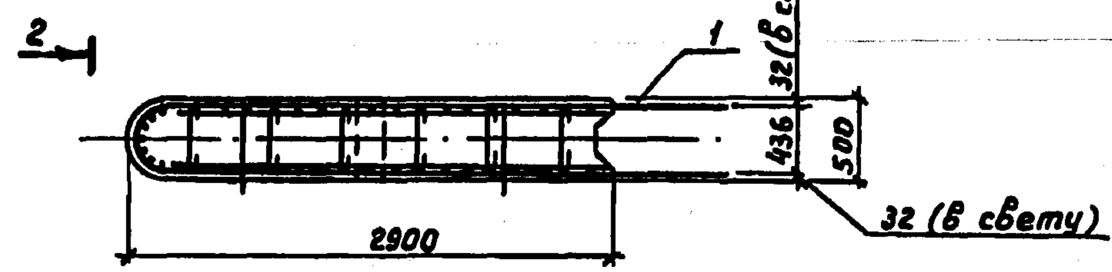
План
