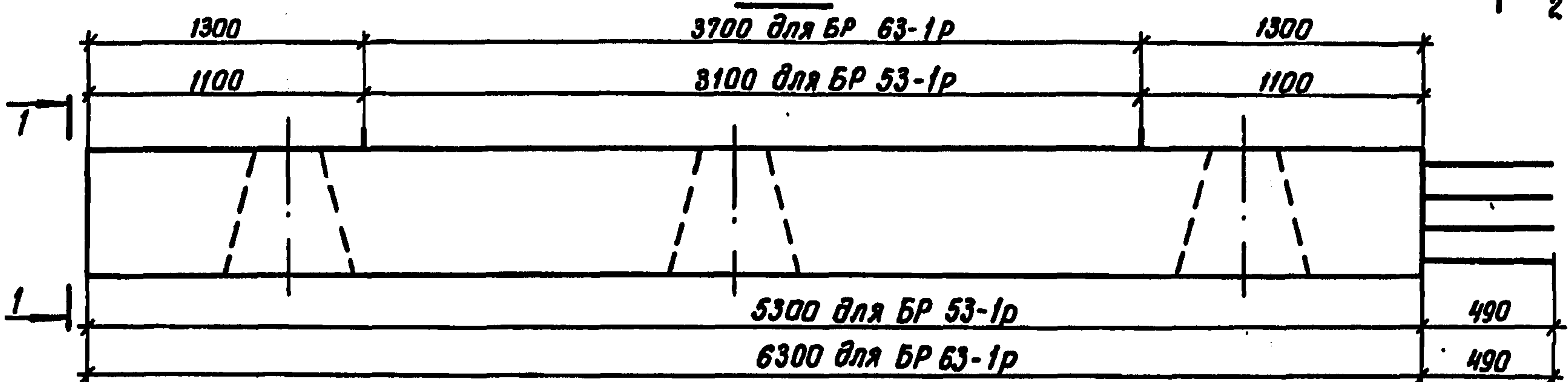
План
