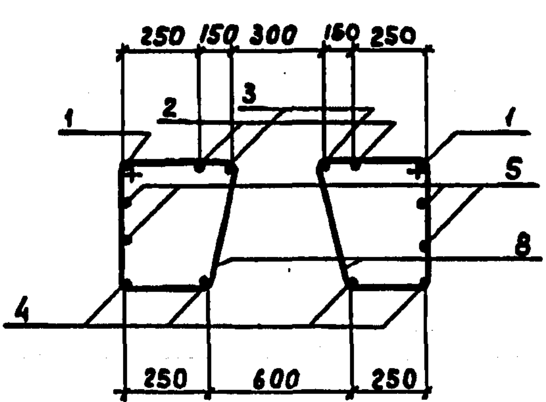
Сечение 2-2
