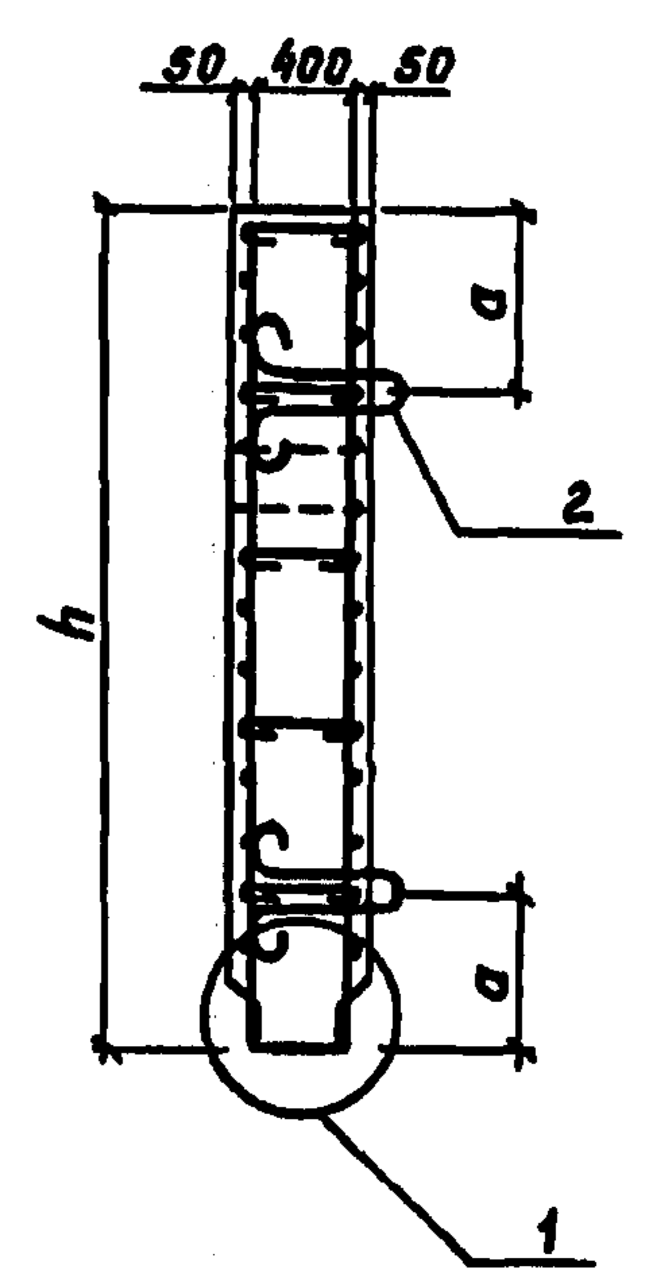
Вид 2-2
