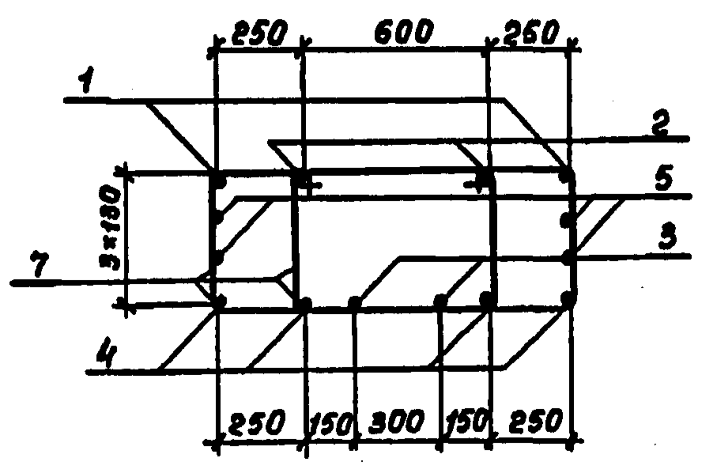
Сечение 1-1
