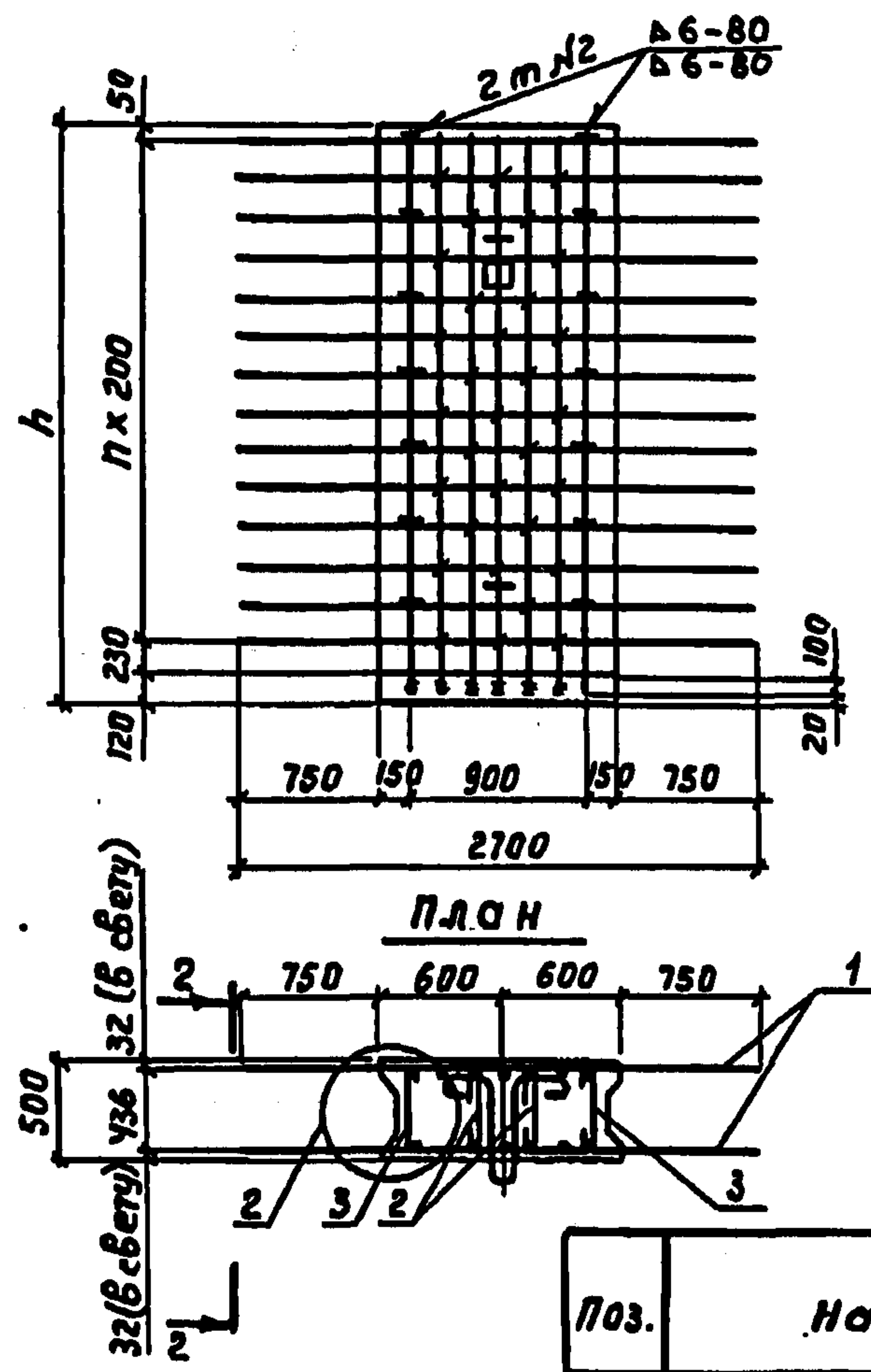
Схема армирования
