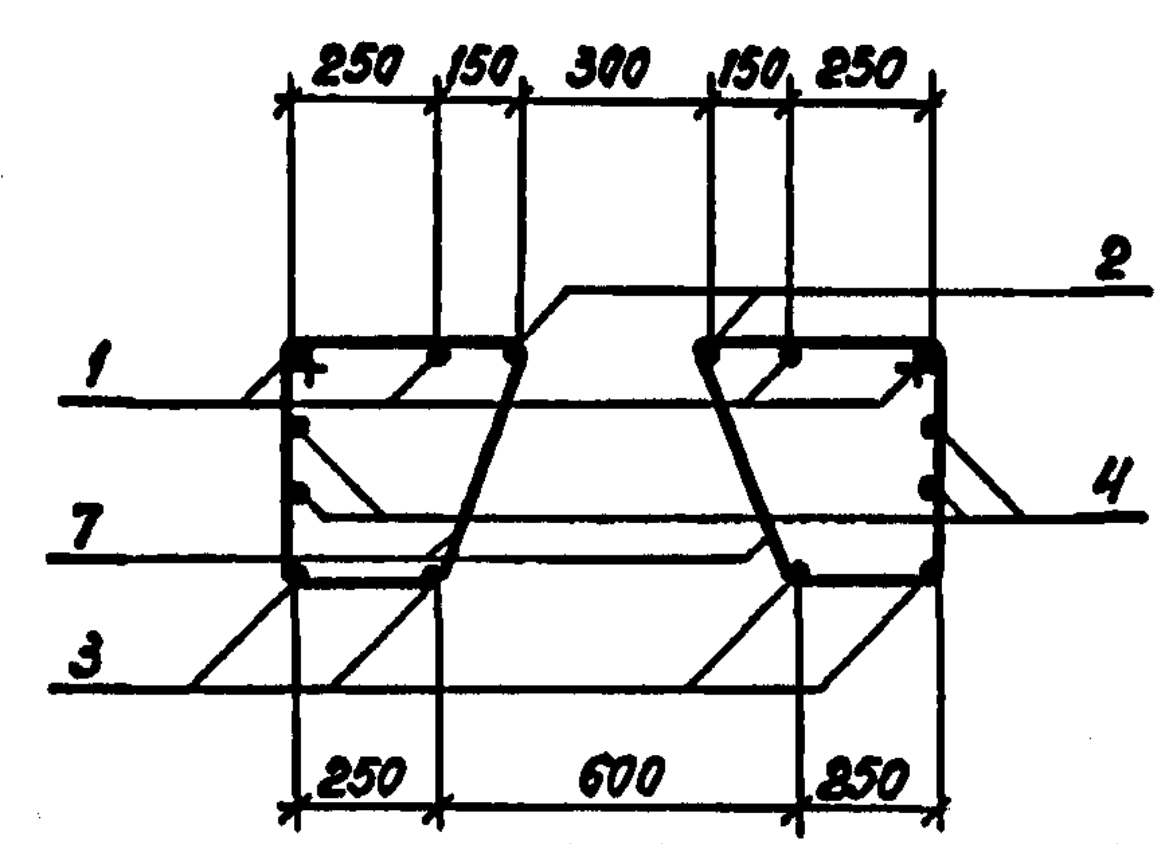
Сечение 2-2
