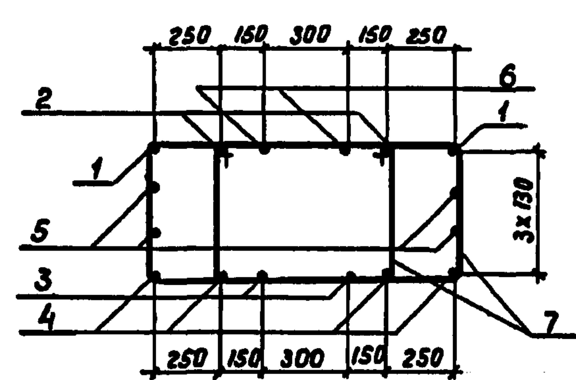
Сечение 3-3 Остальное см. рис. 1
