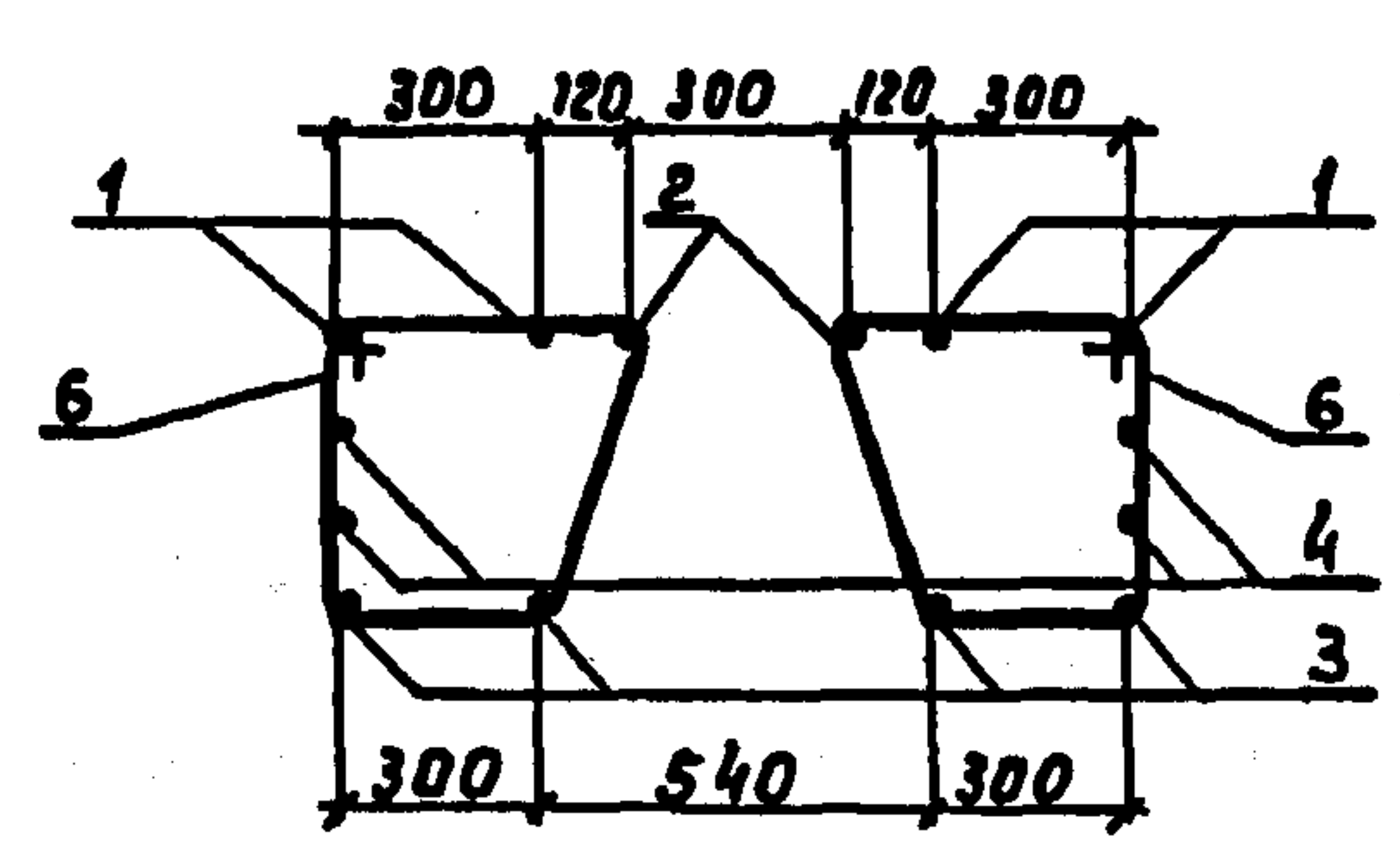
Сечение 2-2
