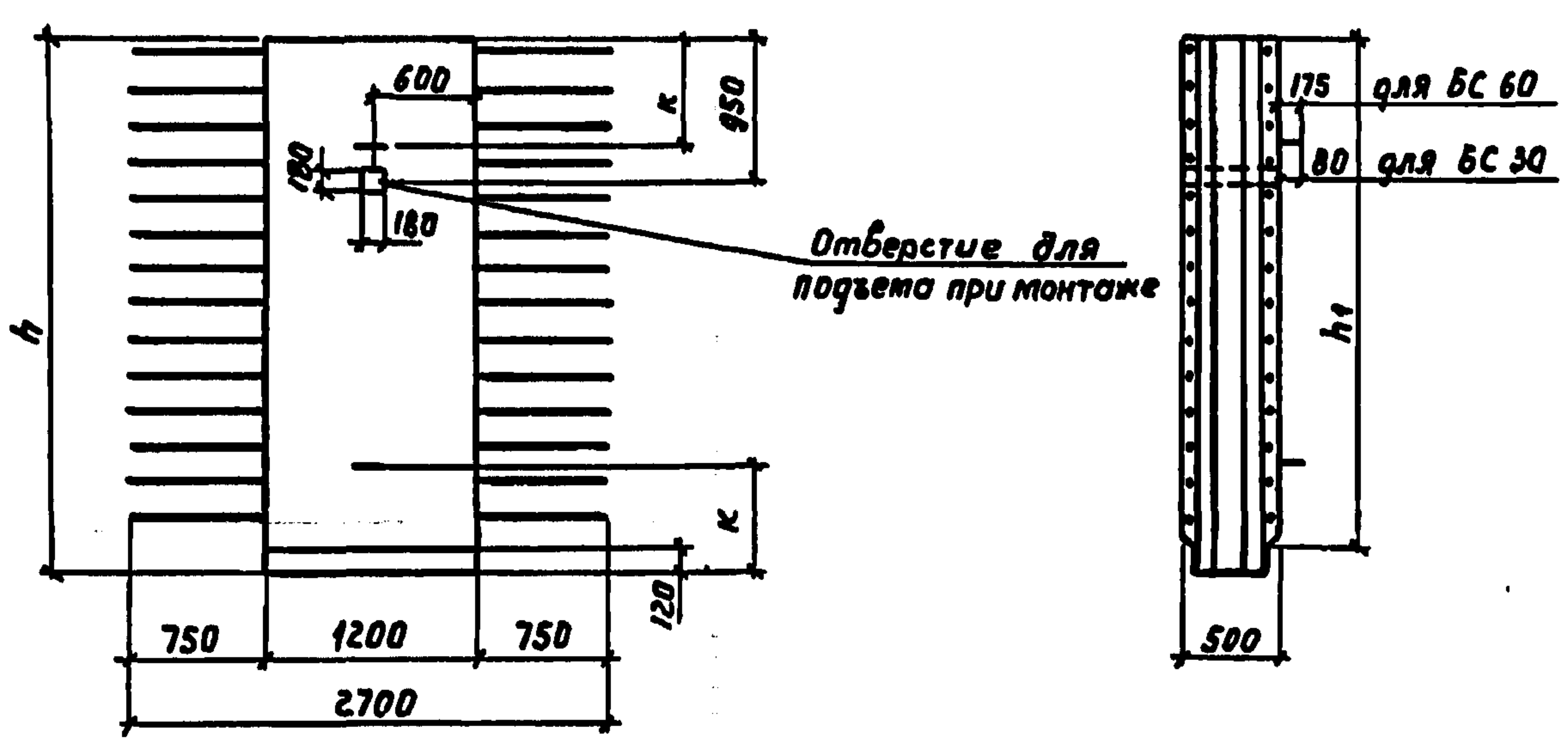
Вид 1-1
