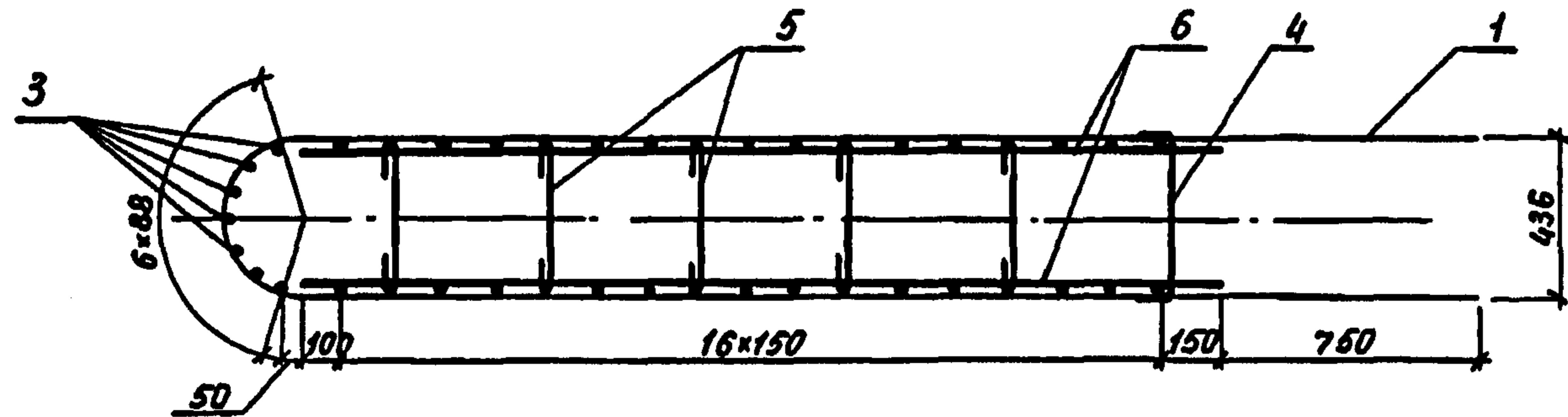
Разрез 1-1
