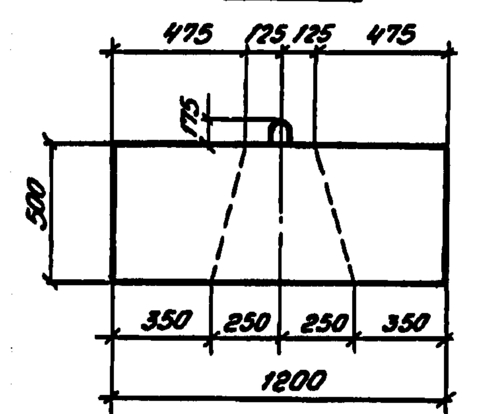
Вид 2-2
