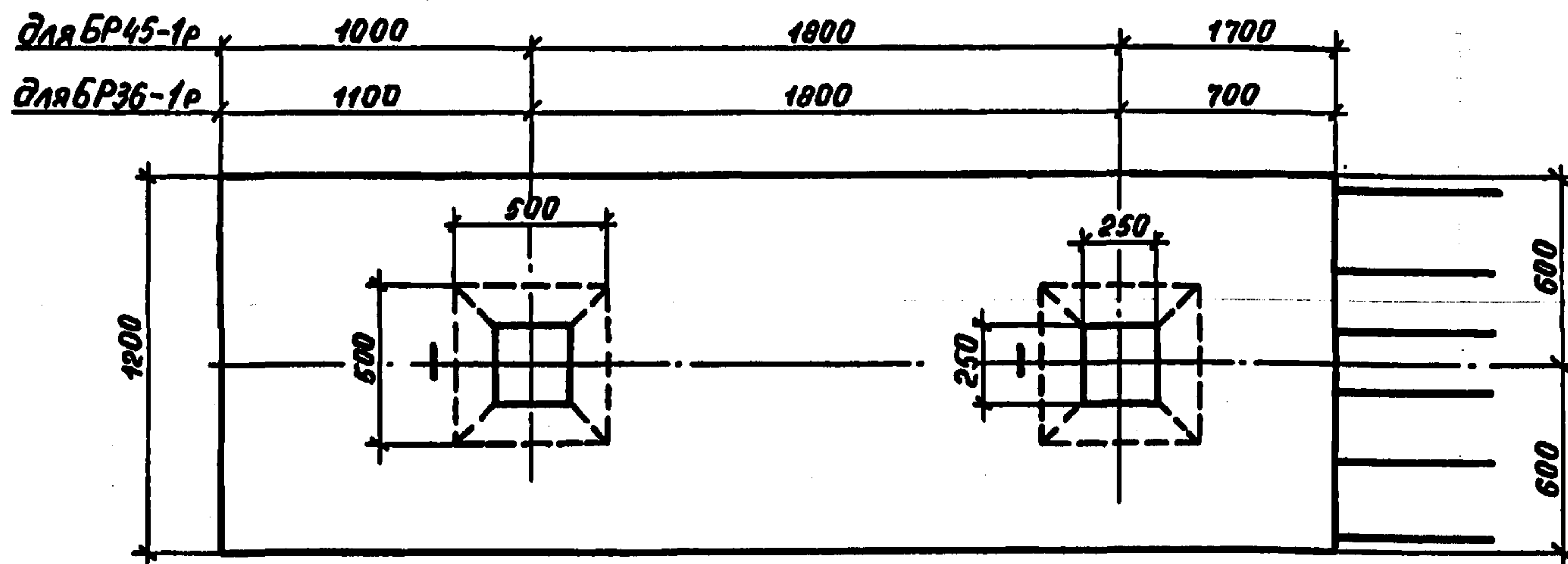
Схема армирования
