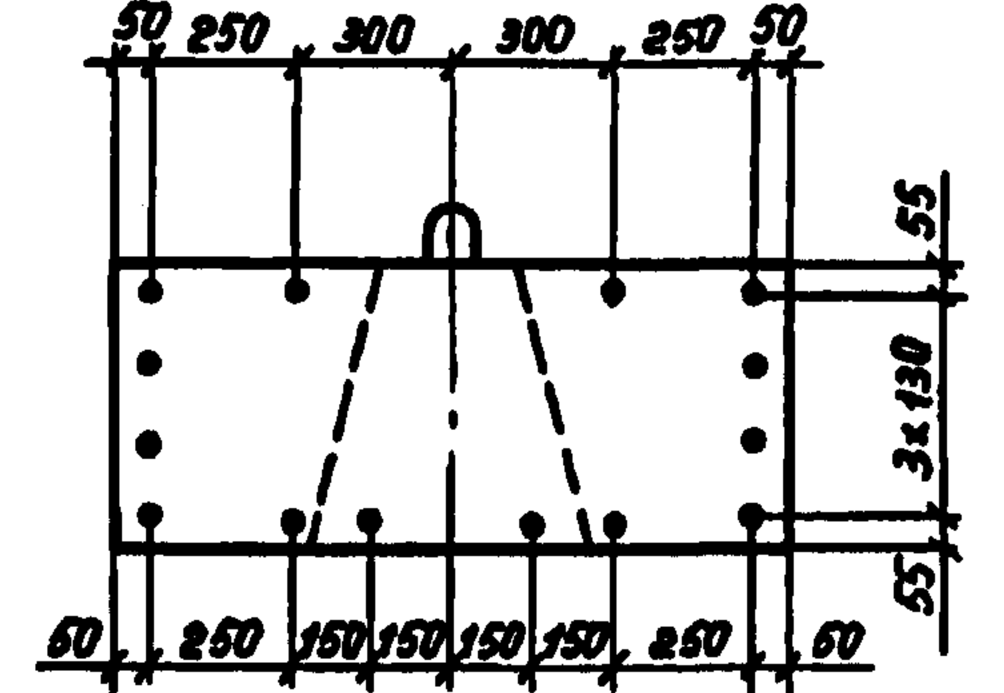
Вид 2-2
