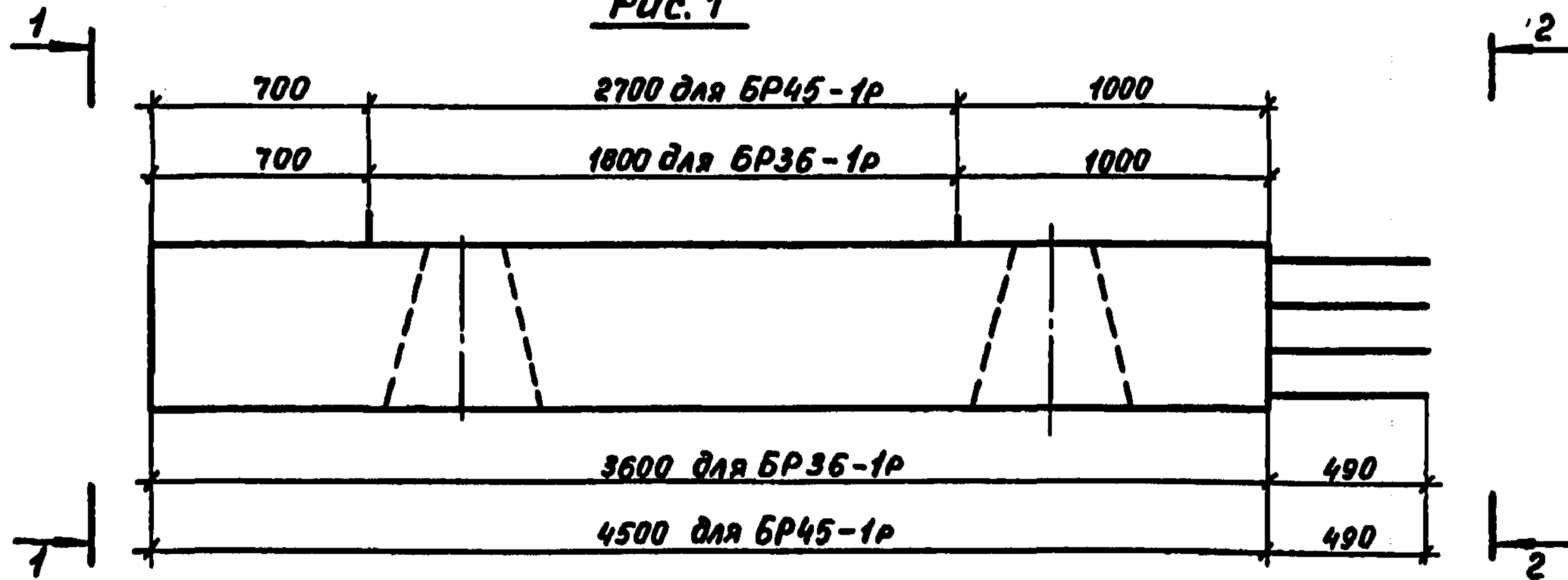
План
