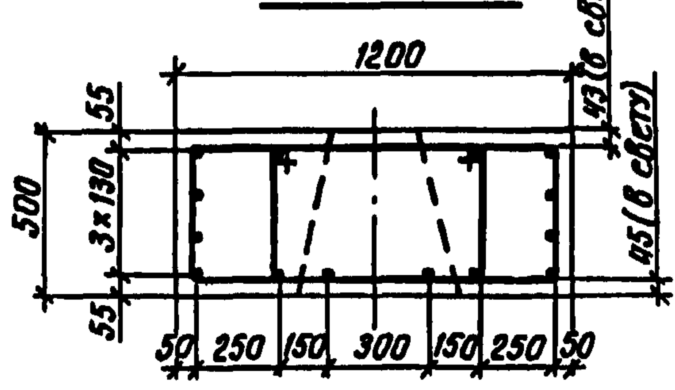
Сечение 3-3
