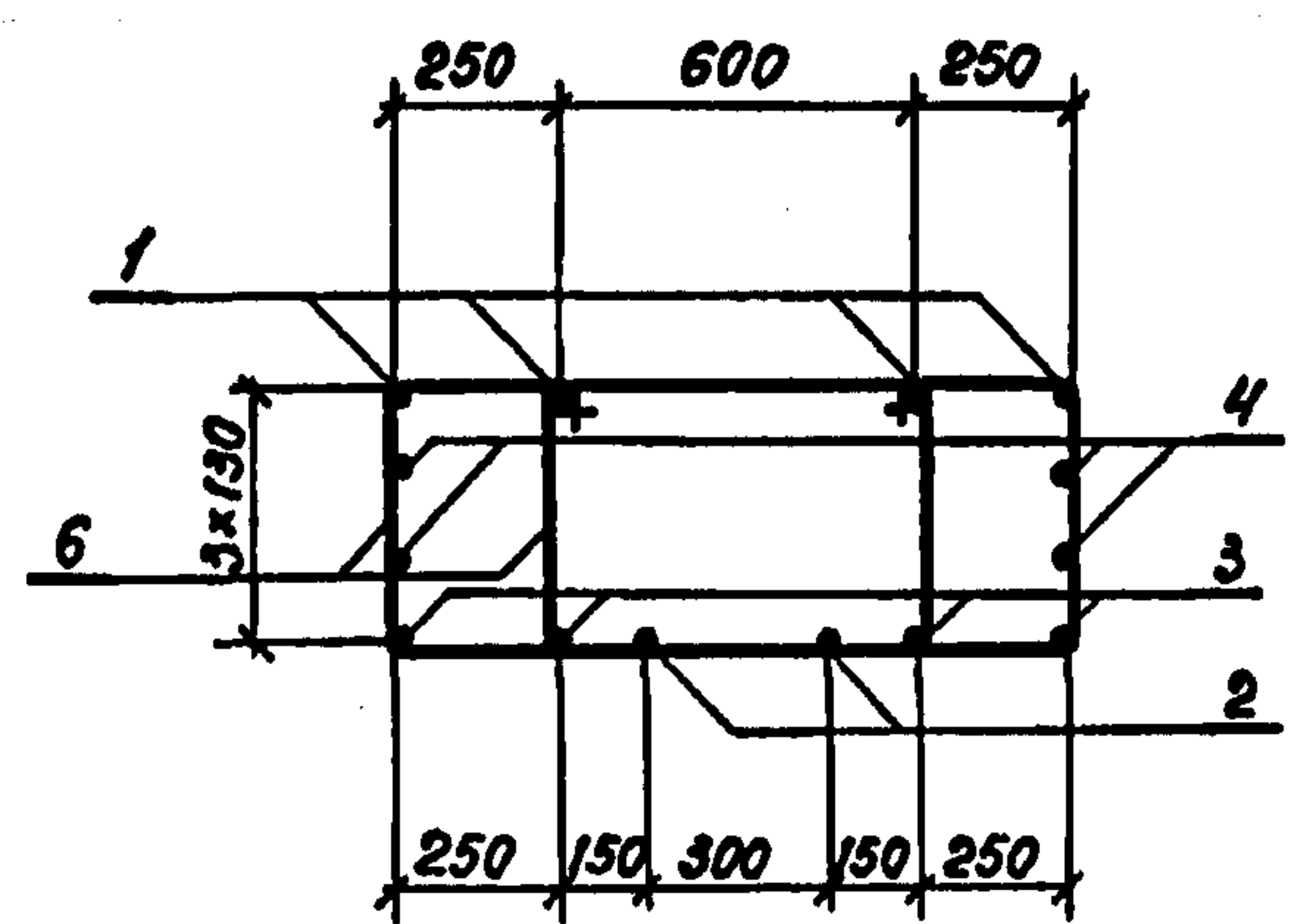
Сечение 1-1
